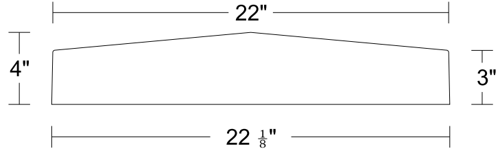
WC507-22.125
