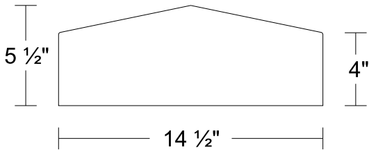
WC507-14.5
