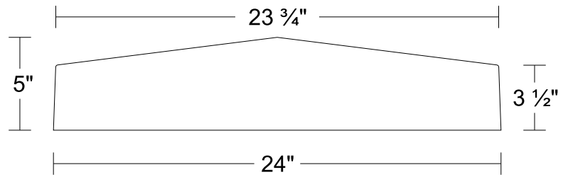
WC507-24x3.5x24
