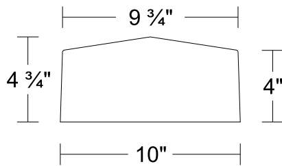
WC507-10x4.75
