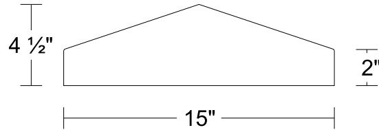
WC507-15x4.5
