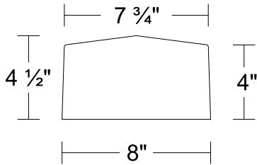
WC507-8x4.5
